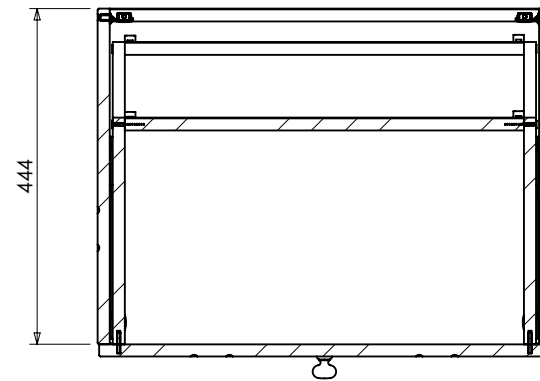
B-B
