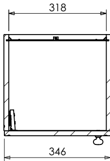
B-B
